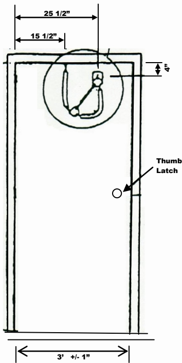
BULKHEAD DOOR
